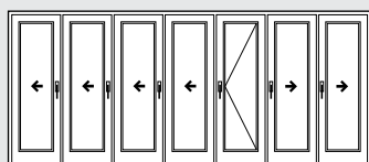
743-as séma 6 harmonika szárny 1 nyílószárny
