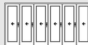
660-as [2] séma 6 harmonika szárny
