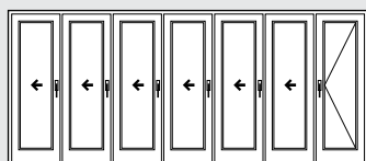
761-es [1] séma 6 harmonika szárny 1 nyílószárny
